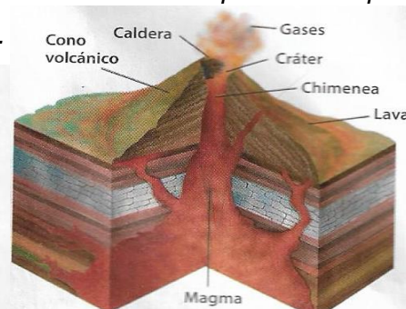
Esquema del interior de un volcán
